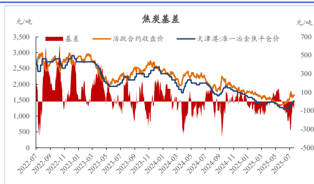
图 19. 焦炭基差
