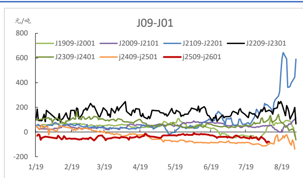
图 21. J2509-J2601 月差
