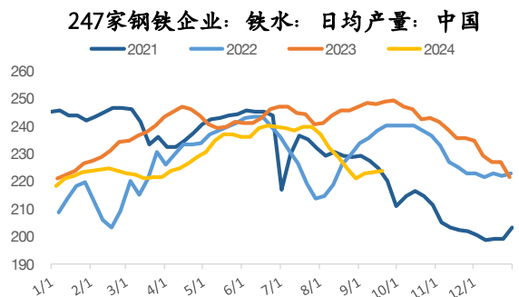
图 10：247 家钢企日均铁水产量
