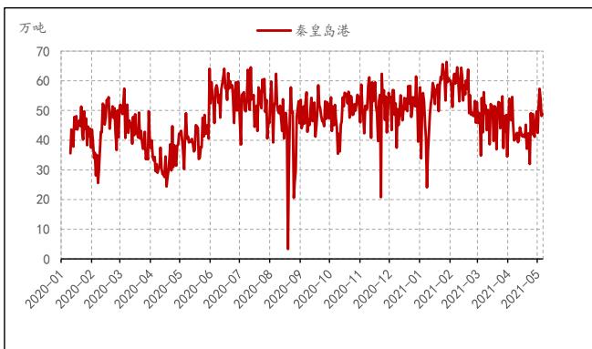
图. 秦皇岛港铁路调入量
