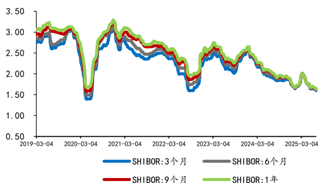
图 44: SHIBOR 利率
