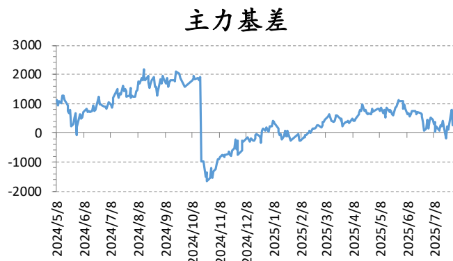
图 12：主力基差
