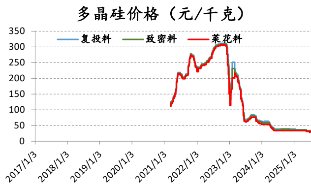
图 7：多晶硅价格
