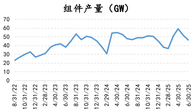
图 21：组件产量
