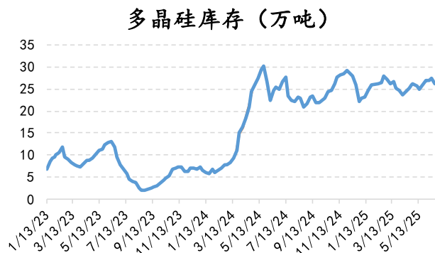
图 16: 多晶硅库存
