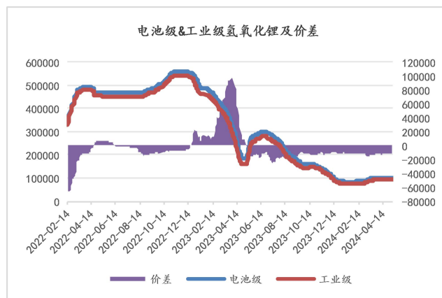
图 5：电池级、工业级氢氧化锂及价差
