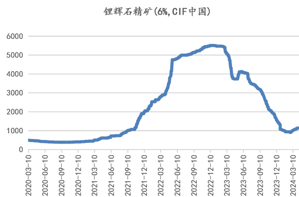
图 7：锂精矿现货价格（SC6, CIF, 美元/吨）
