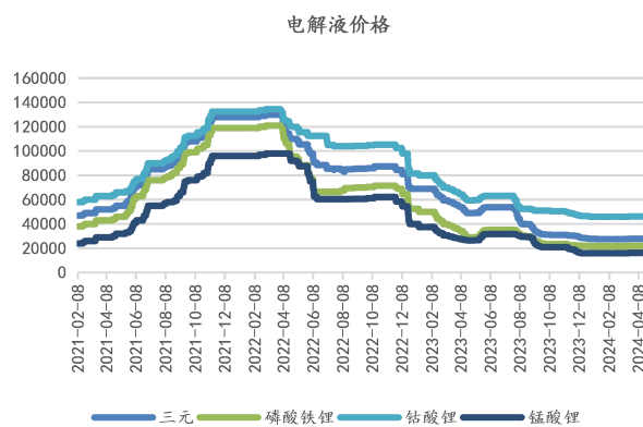
图 11：各电解液价格（元/吨）
