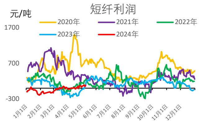
图 13: 短纤利润
