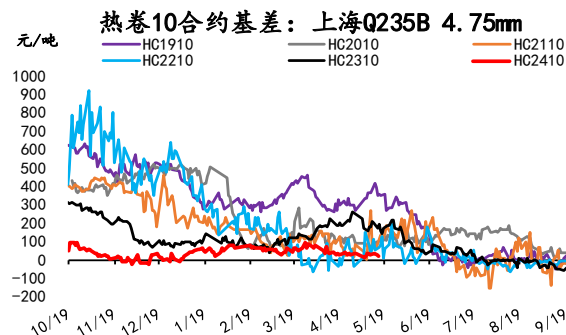
图 44.热卷 10 基差
