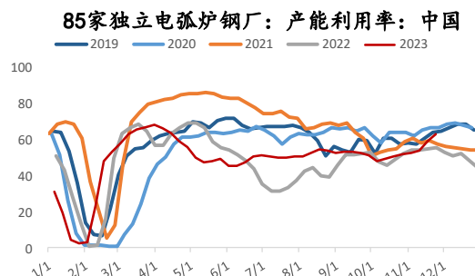
图 28：85 家独立电弧炉钢厂产能利用率
