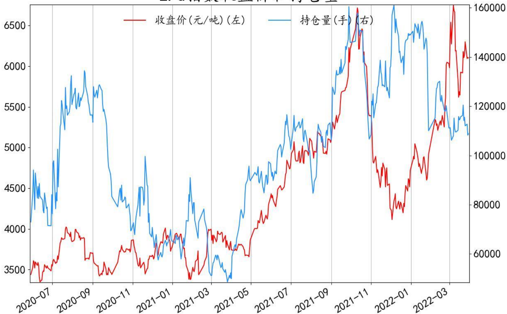
LPG指数收盘价和持仓量
