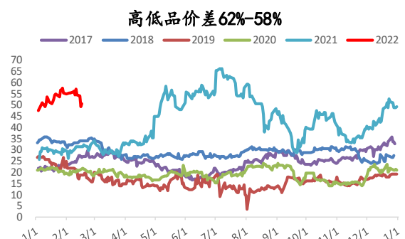
图 18. 高低品价差
