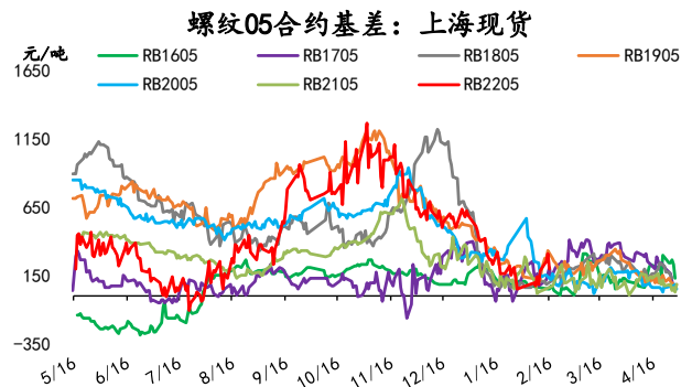
图 41. 螺纹 05 基差
