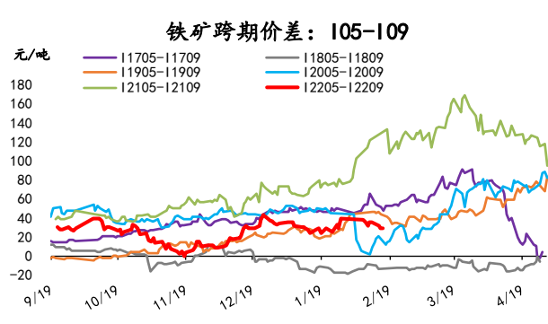
图 16. 铁矿 5-9 价差
