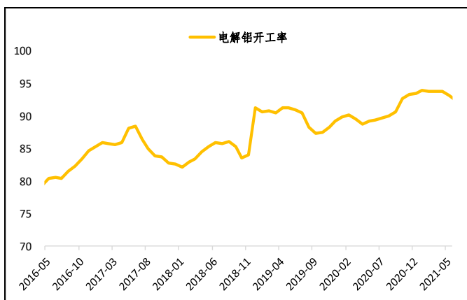
图 14. 铝下游需求 (%)
