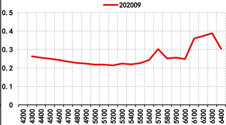
棉花看跌期权隐含波动率
