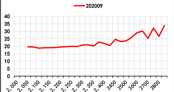
菜粕看跌期权隐含波动率
