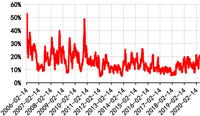
棉花指数20日历史波动率
