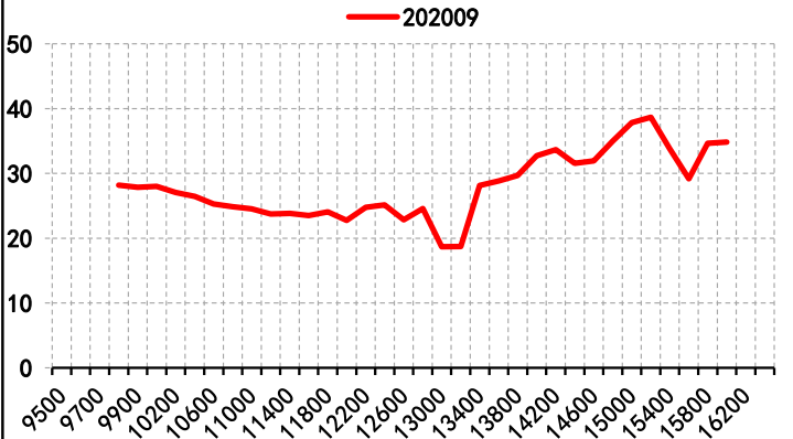
PTA看跌期权隐含波动率
