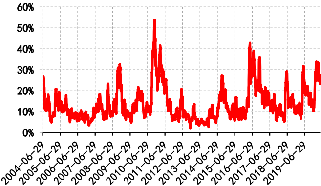
TA指数20日历史波动率
