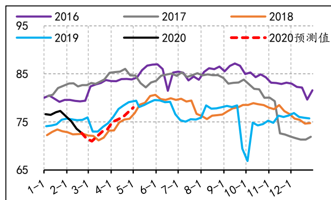
图1：全国163家钢厂高炉产能利用率（万吨）
