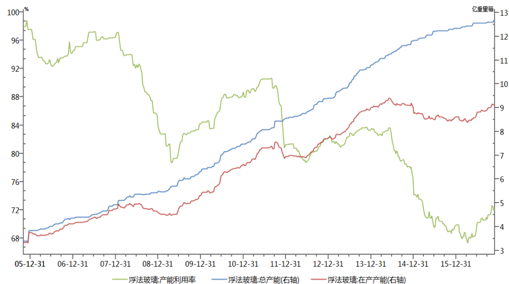
图 22、 浮法玻璃产能、在产产能、产能利用率
