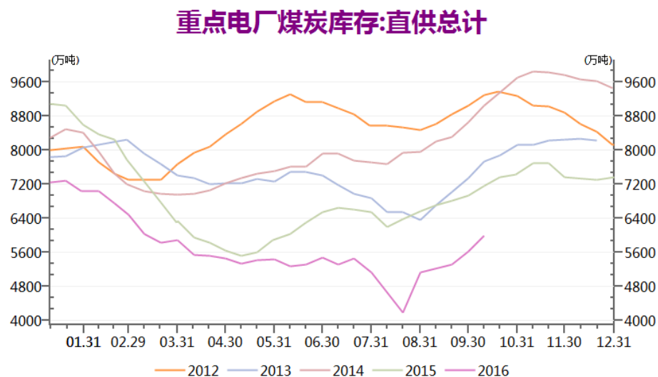
图 15、重点电厂库存
