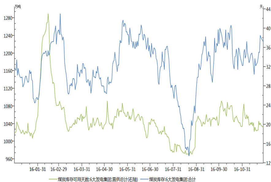
图 12、6大发电集团煤炭库存及可用天数
